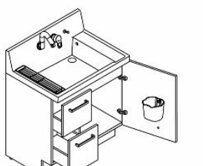
引出タイプ AR3H-755SY/LP2H
