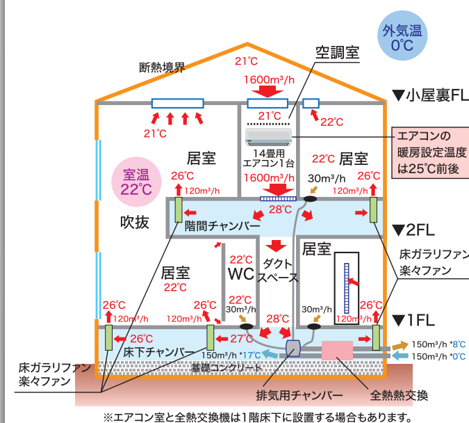
空調スペシャル【暖房時】の空調状況 (イメージ)
