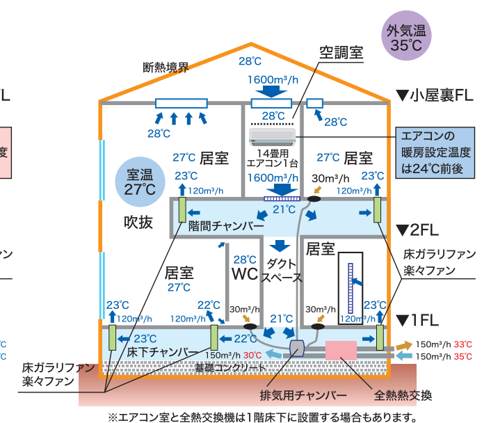
空調スペシャル【冷房時】の空調状況 (イメージ)
